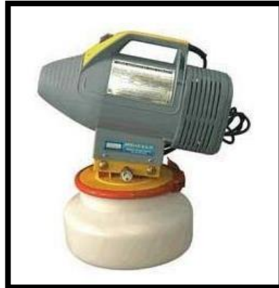
Resim 4. El tipi elektrikli pülverizatör (ULV)
