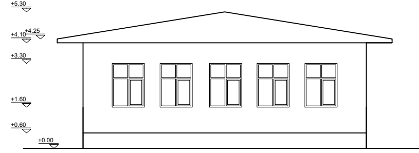
Kuzey-Güney Cepheleri
